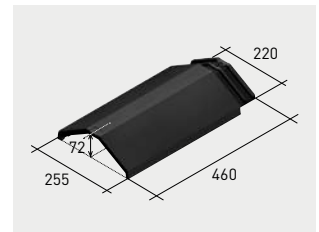
Q120*K | Cumbreira angular klinker
