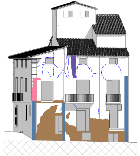
2 Estado previo. Alzado 3 -- 1 : 200
