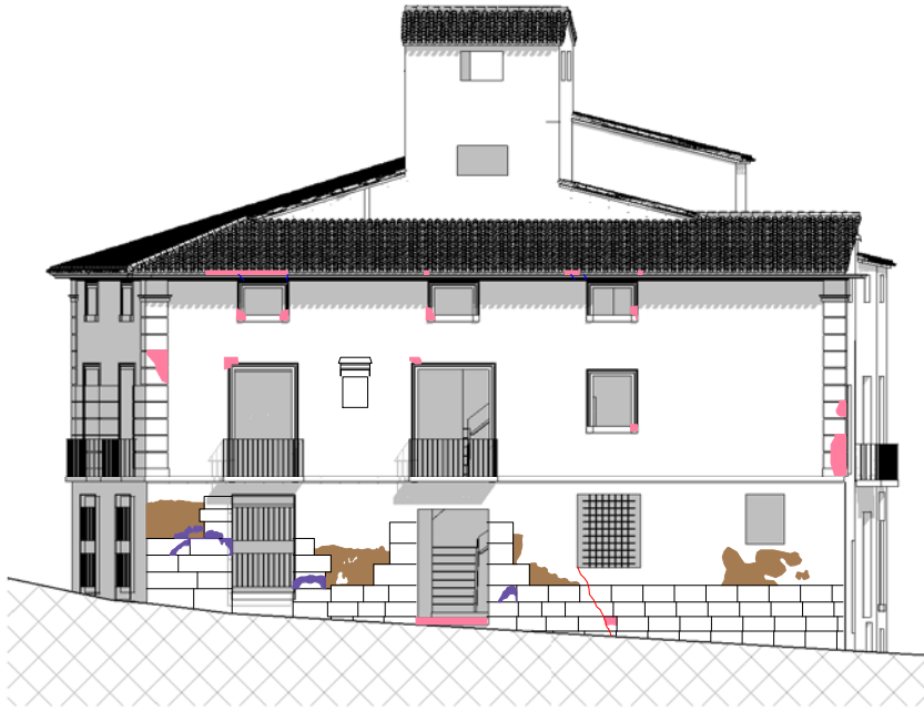
1 Estado previo. Alzado 2 -- 1 : 200
